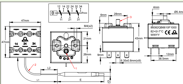
Тип с креплением 2 винтами M4
