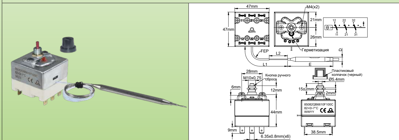
Тип с креплением центральной втулки М10
