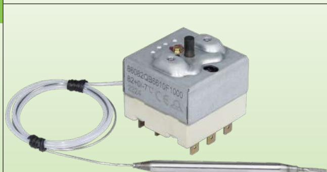
Тип с креплением 2 винтами M4
